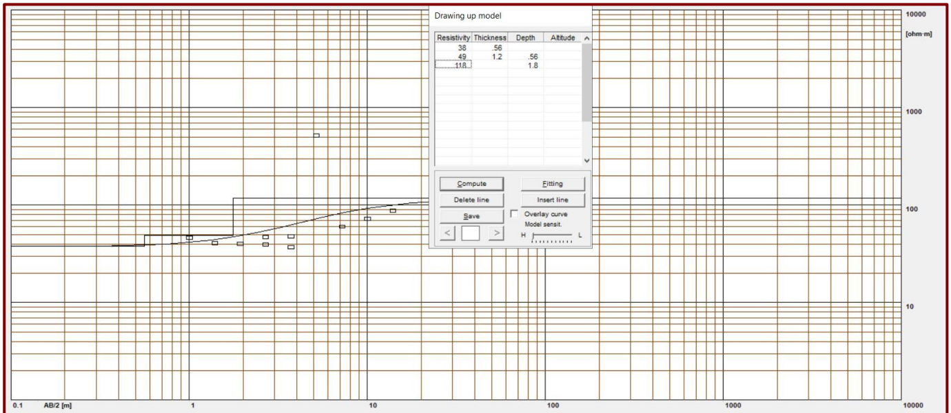
Fig.14a - Graphe géo-électrique du SE1
