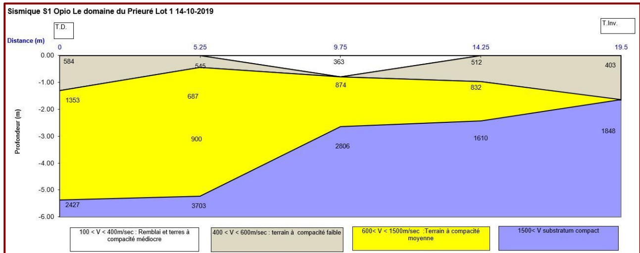
Fig.12 - Coupe sismique S1
