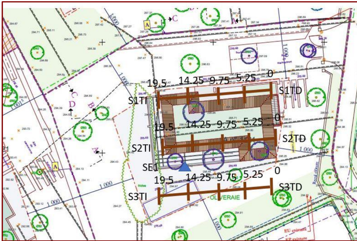
Fig.11 : Implantation des mesures géophysiques
